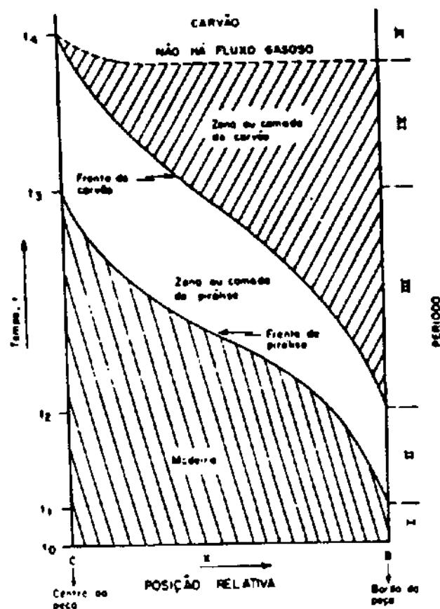
Figura 3.1 - Diagrama de carbonização proposto por Kanury e Blackshear (apud Oliveira et al., 1982)
