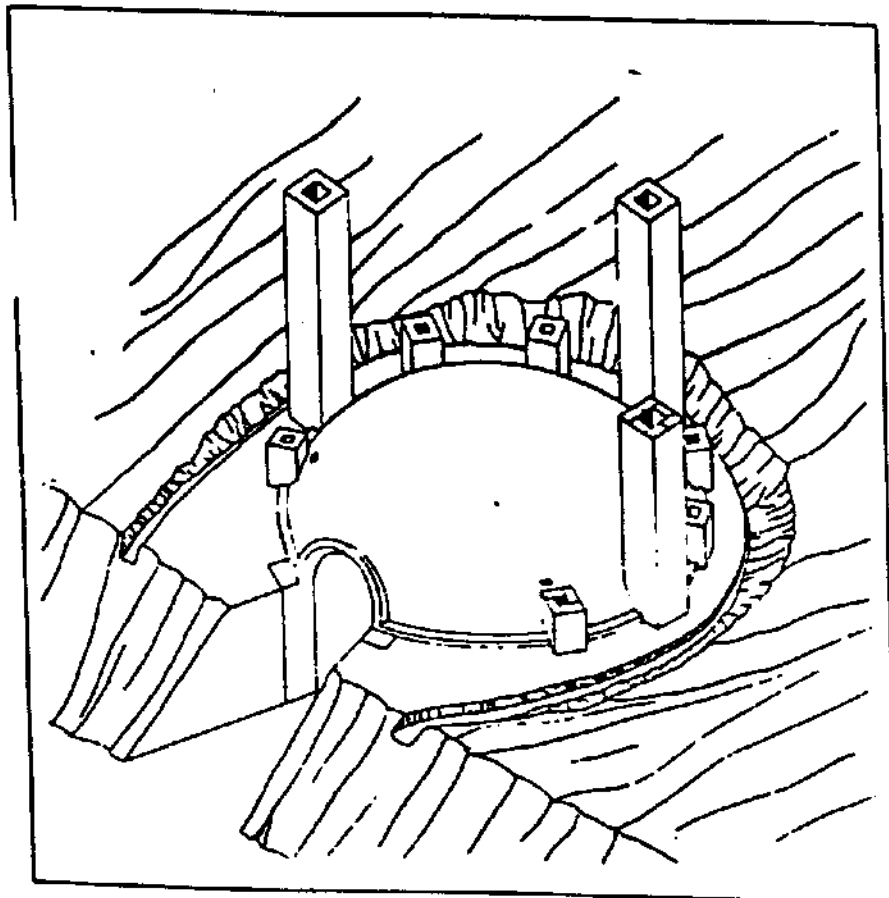
- Figura 3.14 - Ilustração do forno de encosta
