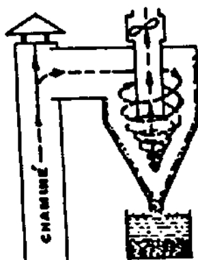
Figura 3.10 - Diagrama do recuperador de alcatrão "tipo ciclônico"
