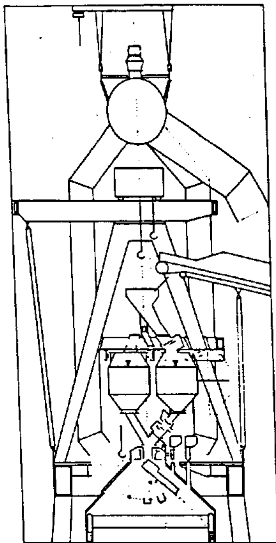
Figura 3.12 - Ilustração do sistema de carregamento Paul Wurth
